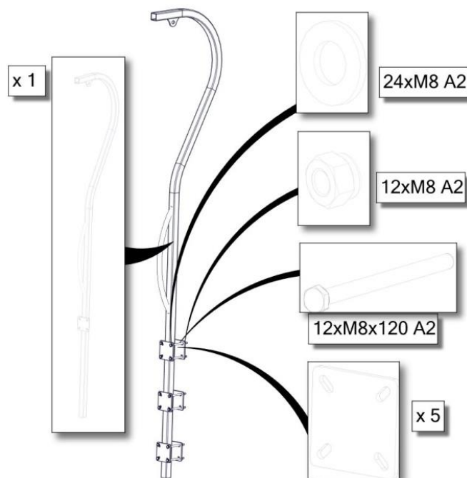
Rysunek 2. Zestaw montażowy AT165B
