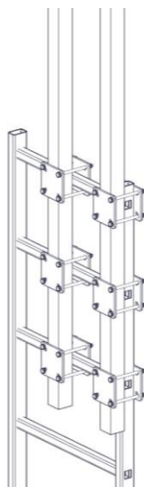
Rysunek 5. Sposoby objęcia szczelki i pobocznic drabiny
