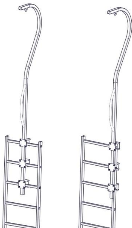
Rysunek 4. Instalacja punktu kotwiczenia do pobocznic drabiny oraz do szczelki drabiny
